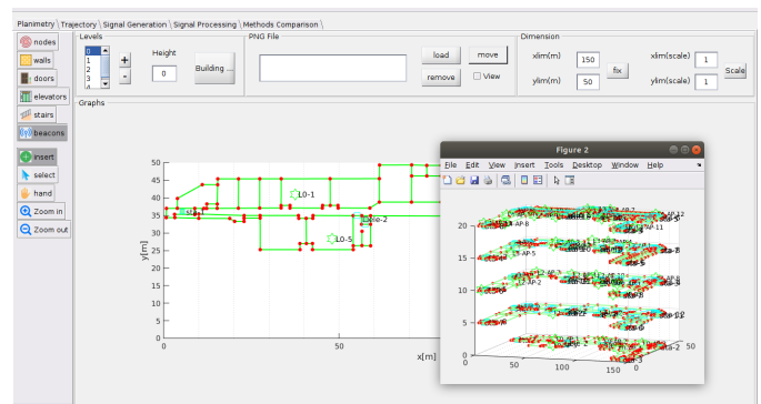
Figura 2. Interfaz gráfica para el diseño de la planimetría building . En la imagen se muestra la interfaz con un edificio de cinco plantas. La figura externa es una representación tridimensional del edificio.
